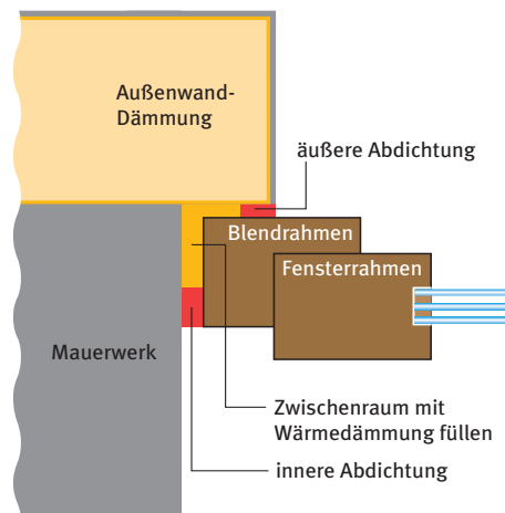
Einbausituation Fenster bei gedämmter Außenwand
